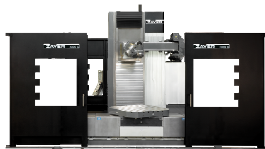
Centro de mecanizado de bancada fija con mesa giratoria Bed type machining center with rotary table
